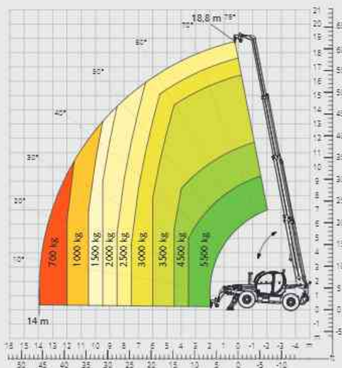
Esquema de capacidades de carga con GANCHO 6000 kg ATT-05-001
